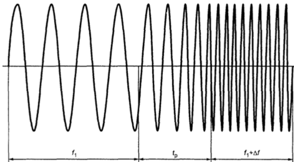
Рисунок 2. Пример изменения частоты в течении переходного интервала времени t_p
